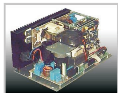
Gleichrichter als Modul
